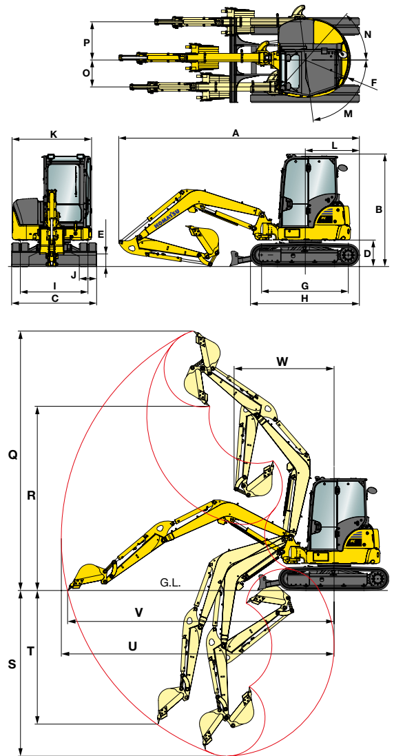
PC35MR-5, cabina, pattini in gomma, lama abbassata, benna da 80 kg
